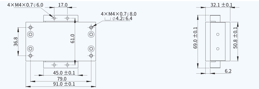
尺寸图
